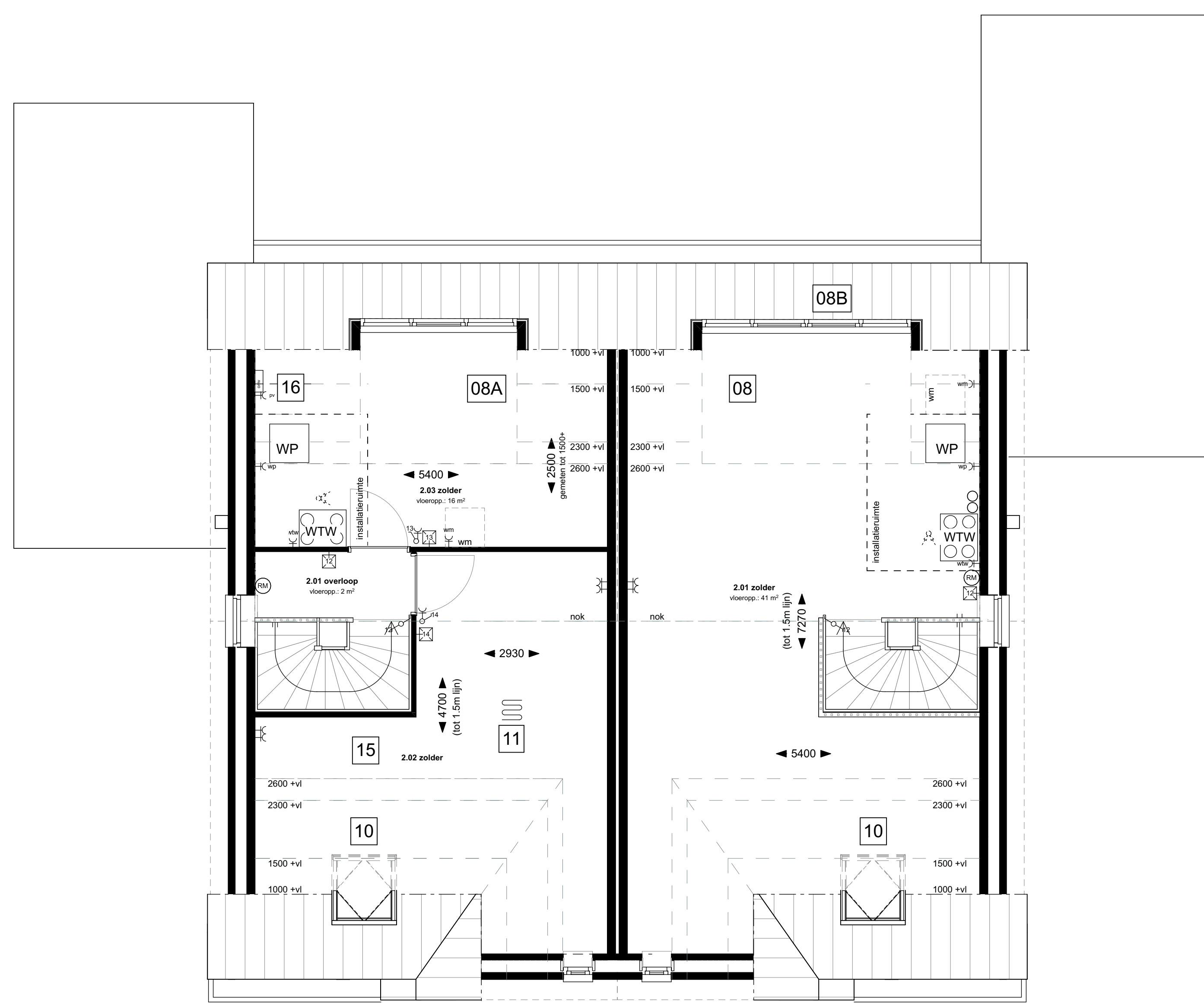
2e VERDIEPING
