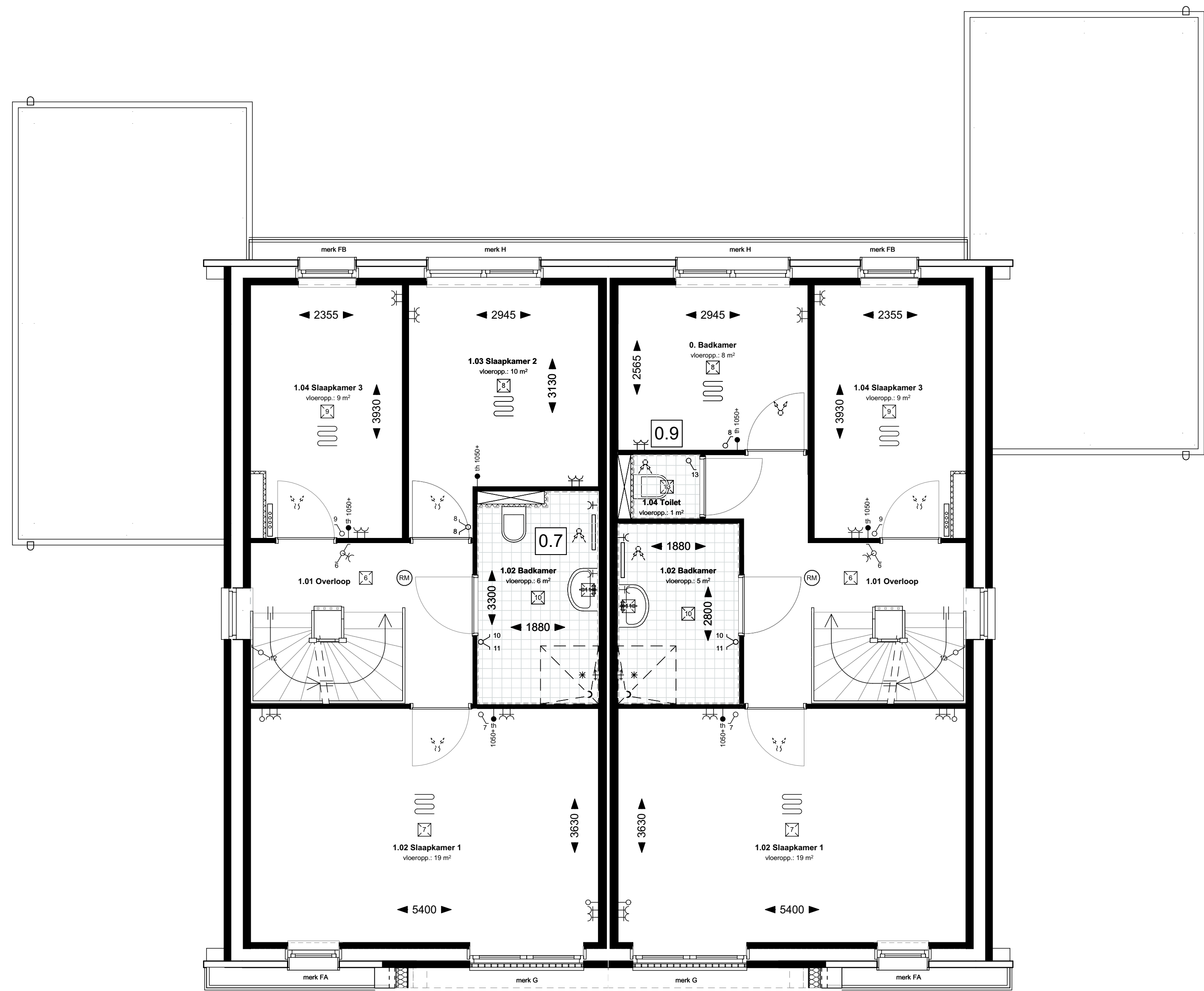
1e VERDIEPING
